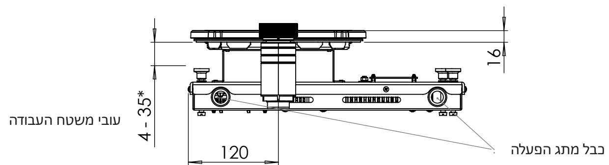
מבט חזיתי
