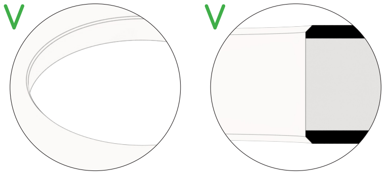
יש לבצע חיתוך מינימלי (פאזה) של 1 × 1 מ"מ בקצוות העליונים והתחתונים של החתך.
