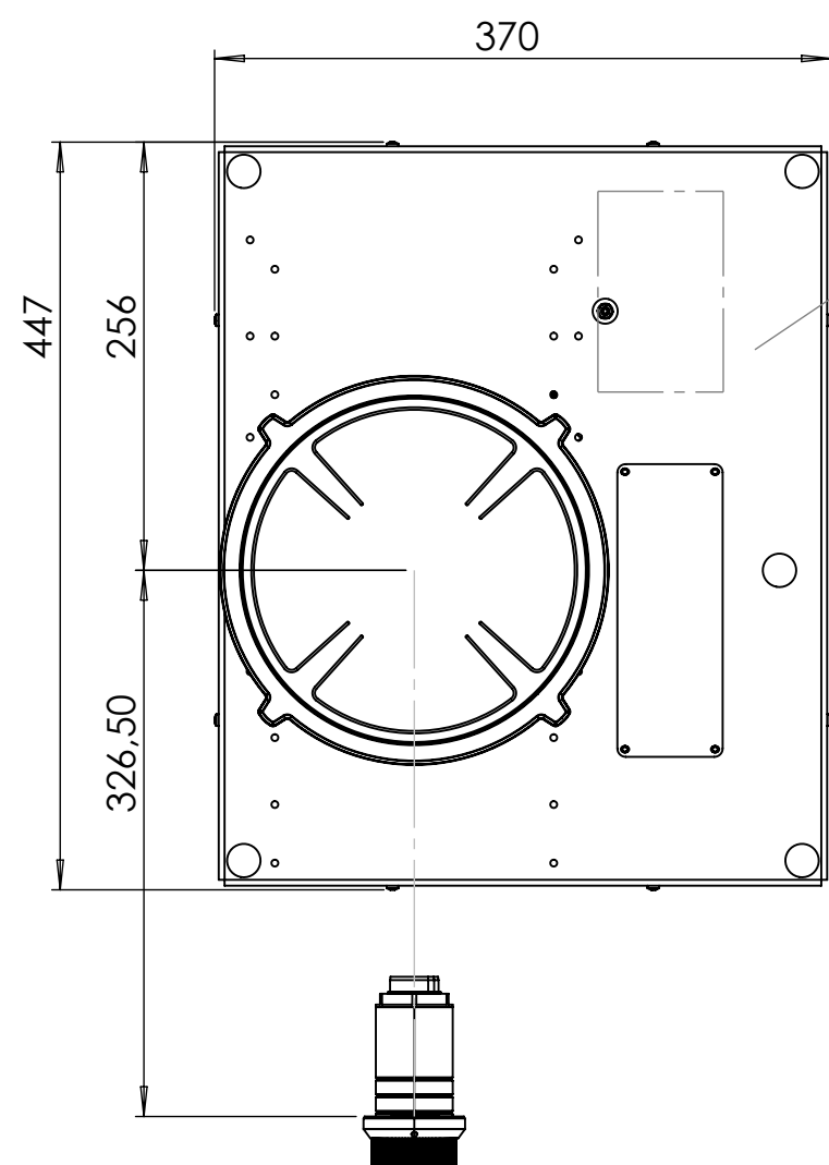
מבט עליון
