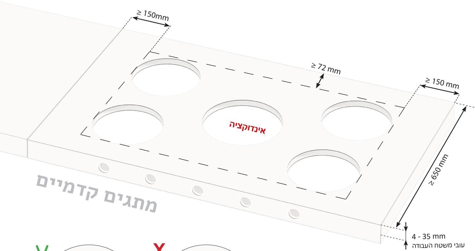
יש לבצע חיתוך מינימלי (פאזה) של 1 × 1 מ"מ בקצוות העליונים והתחתונים של החתך.
