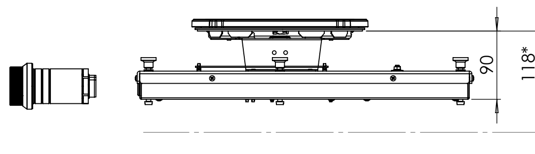
מבט צדדי
