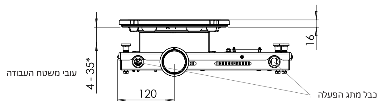
מבט חזיתי
