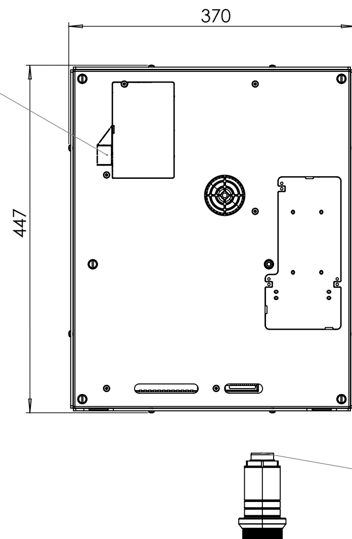
מבט תחתון
